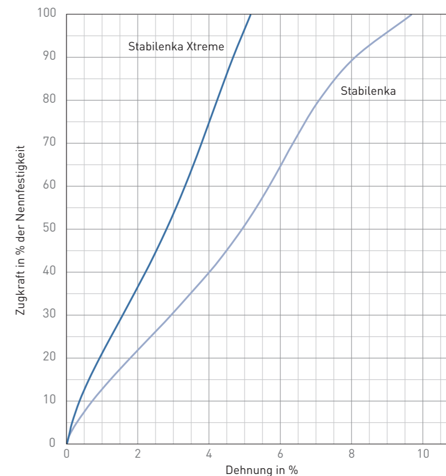
Exemplarische Kurzzeitzugkraft-Dehnungs-Kurven
